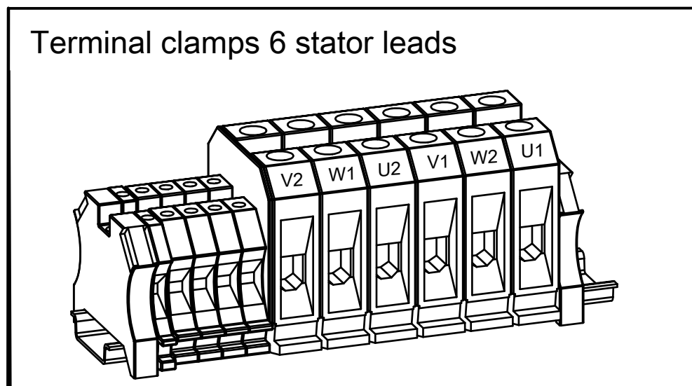
Figura 13: Sujeciones del terminal, 6 conductores del estátor
