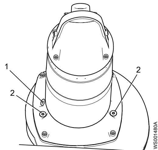
Figura 35: Sin camisa de refrigeración
