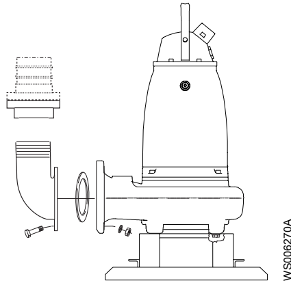
Figura 5: Instalación en S
