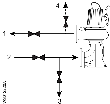
Figura 8: Válvulas de cierre y de ventilación (se muestra una bomba genérica)
