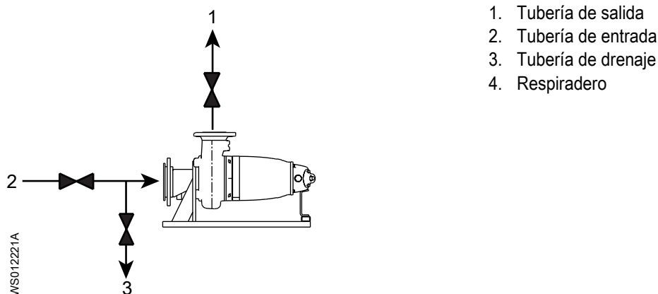
Figura 7: Válvulas de cierre y de ventilación (se muestra una bomba genérica)
