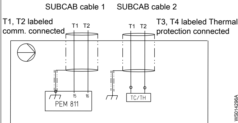
Figura 32: Dos cables SUBCAB™
