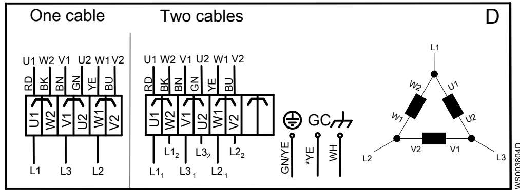
Figura 15: Conexión en D
