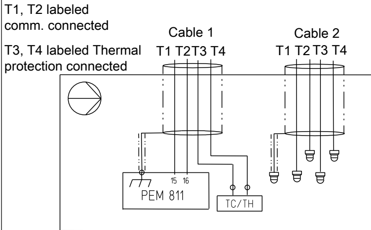
Figura 31: Uno o dos cables SUBCAB™ blindados
