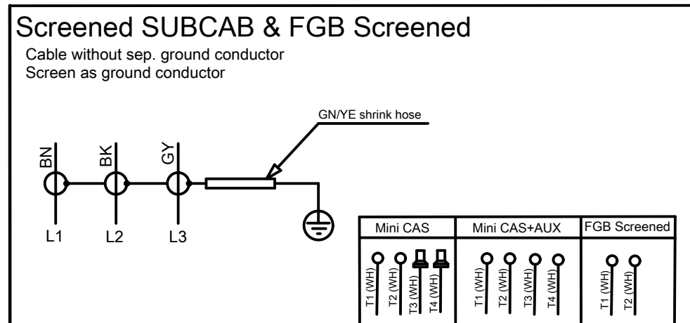
Figura 20: SUBCAB blindado y FGB blindado
