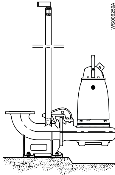
Figura 4: Instalación en P
