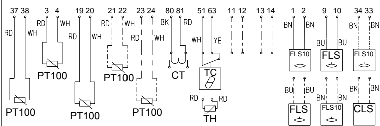
Figura 25: PEM 811 descripción general de la conexión de terminales
