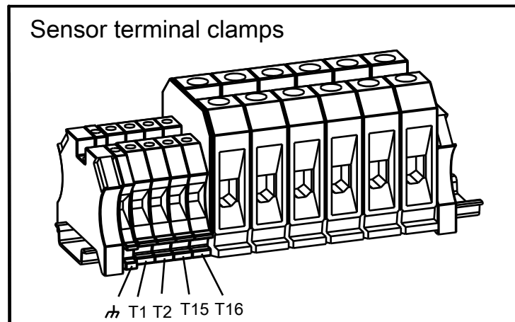
Figura 23: Sujeciones del terminal del sensor
