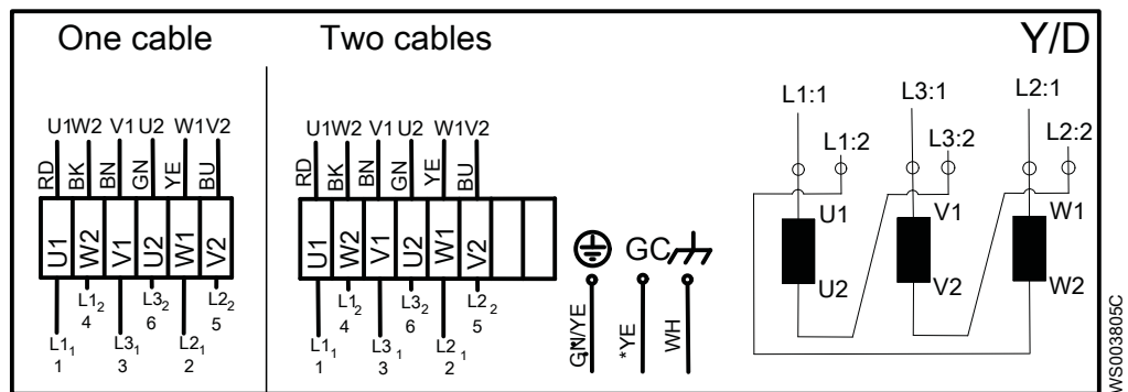
Figura 16: Conexión en Y/D
