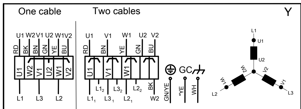
Figura 14: Conexión en Y
