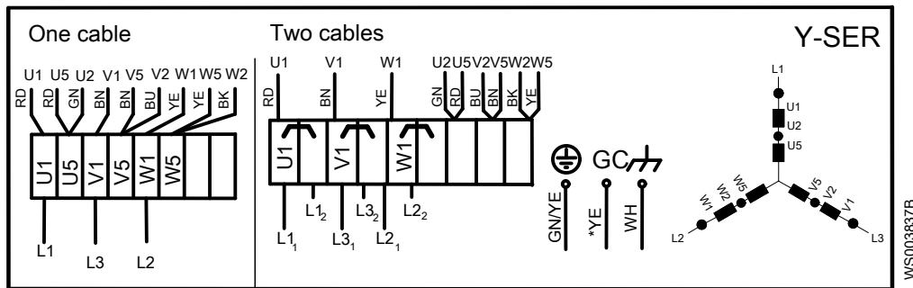
Figura 19: Conexión en Y serie
