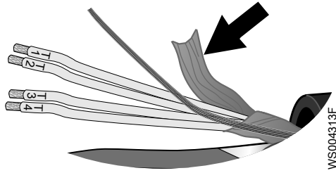
Figura 11: Lámina de aluminio en el elemento de control.
