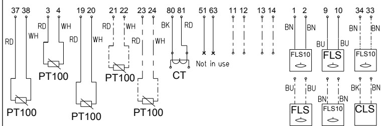
Figura 30: PEM 811 descripción general de la conexión de terminales
