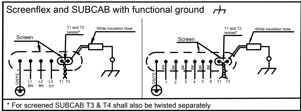
Figura 21: Screenflex y SUBCAB con toma de tierra funcional
