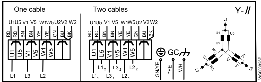
Figura 18: Conexión en Y paralelo
