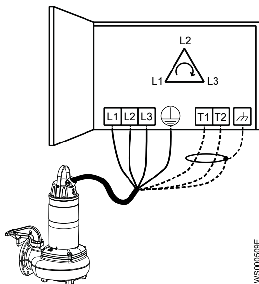
Figura 12: Secuencia de fase
