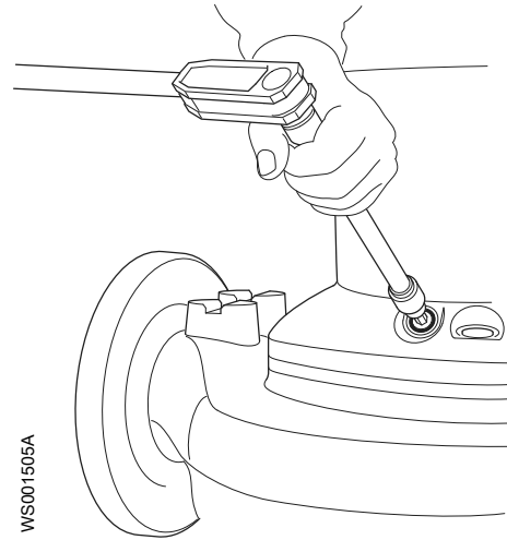
Figura 37: Sin camisa de refrigeración
