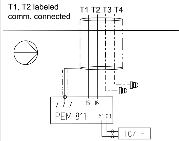
Figura 26: Un solo cable
