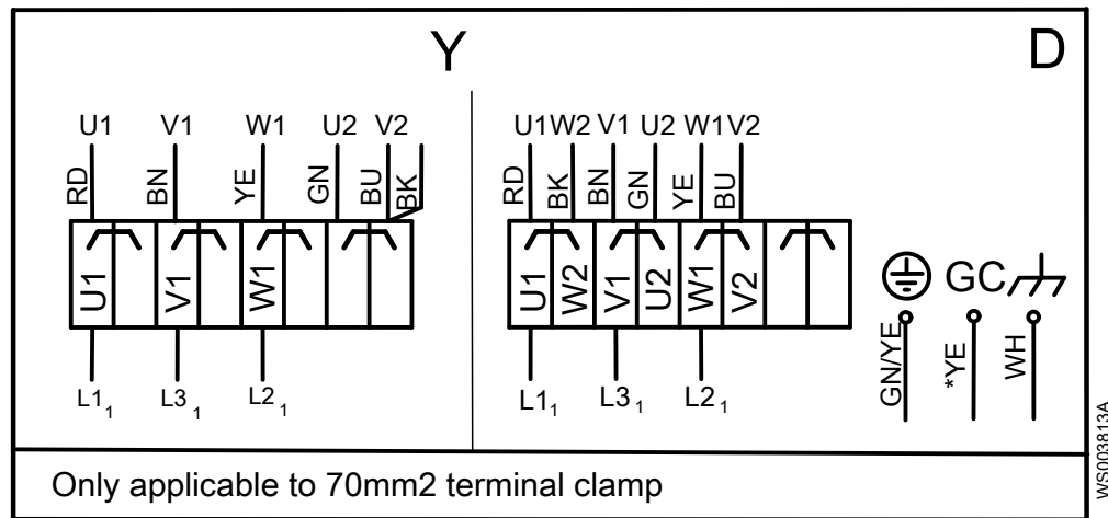
Figura 17: Conexión en Y o D
