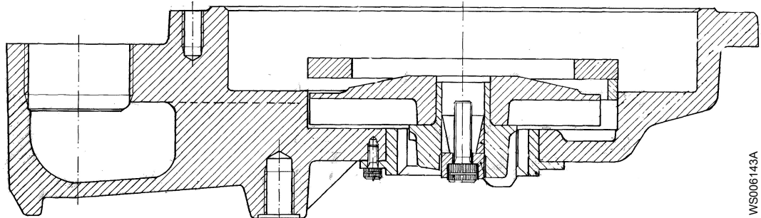
Figura 21: Impulsor M
