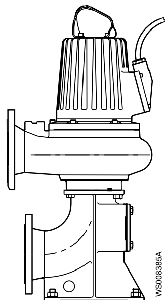
Figura 8: Instalación T
