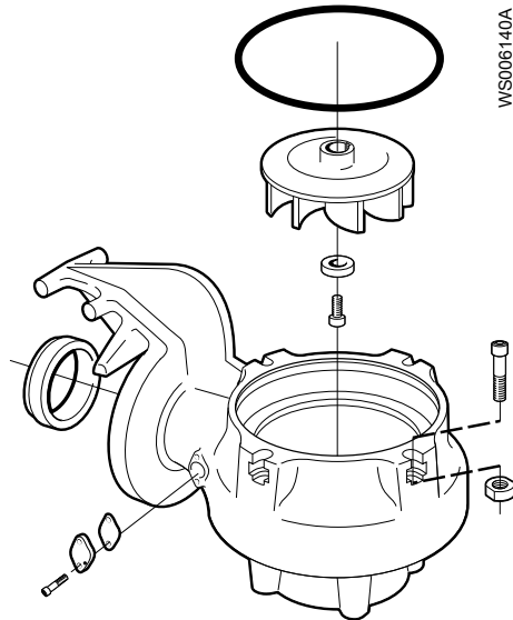
Figura 18: Impulsor D
