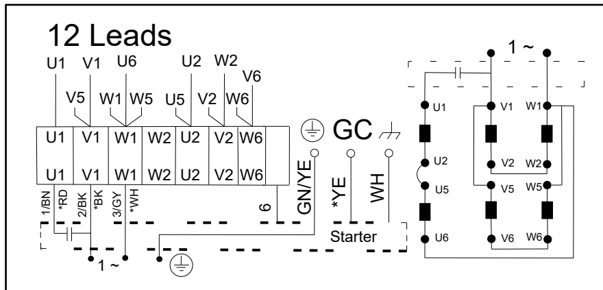
Figura 16: Sin motor de arranque incorporado
