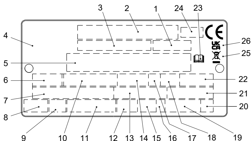
Figura 1: Placa de características
