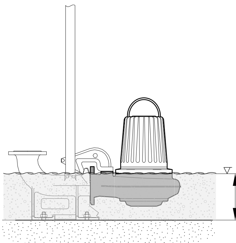
Figura 11: Nivel de agua mínimo
