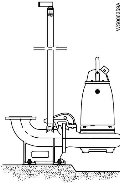
Figura 4: Instalación en P
