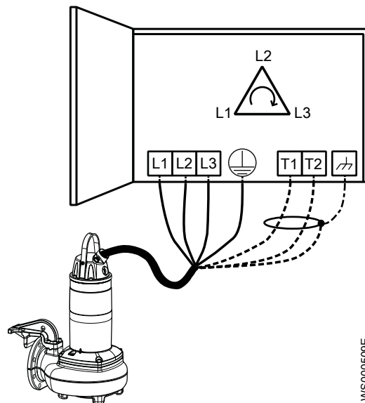
Figura 8: Secuencia de fase
