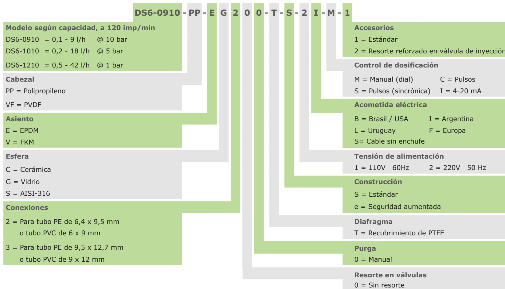
Figura 2 La codificación de la bomba dosificadora se genera a partir de la combinación de las distintas características que se muestran en la figura. No todas las combinaciones son posibles. Consulte por el modelo disponible según las necesidades de la aplicación.
